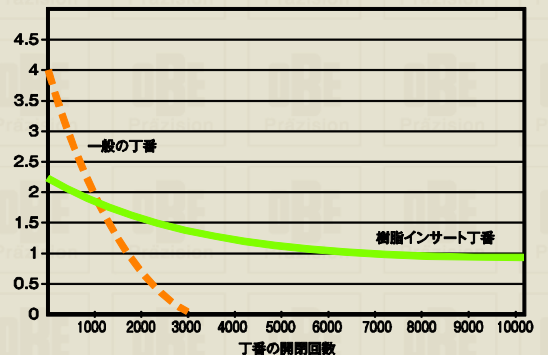
丁番開閉時のアガキ (Nom)
